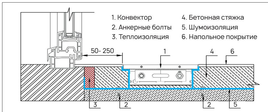
Сечение монтажа внутрипольного конвектора
